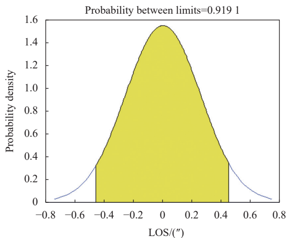
(b) 权重 1 : 2 : 10 满足指标的概率
