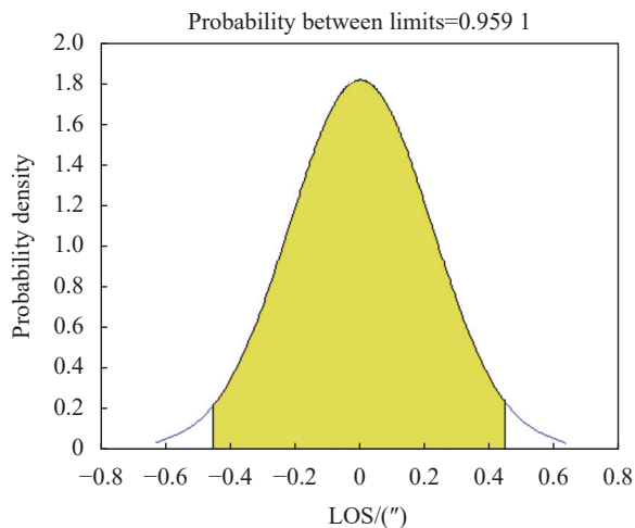
(c) 权重 1 : 2 : 5 满足指标的概率
