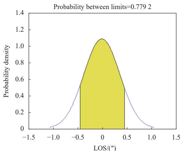
(a) 权重 1 : 2 : 20 满足指标的概率
