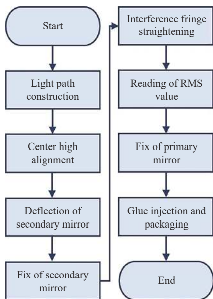
图 12 系统装调步骤
