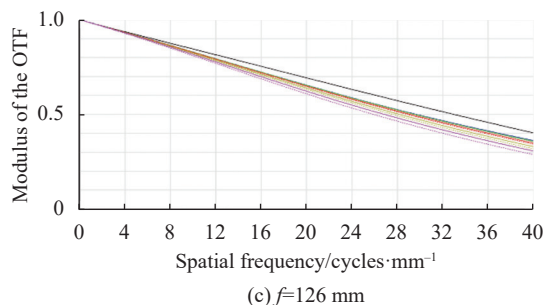
图 5 连续变焦光学系统 MTF 曲线
