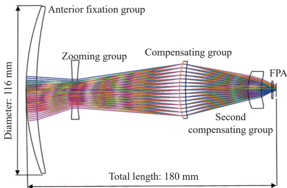
图 4 连续变焦光学系统布局图
