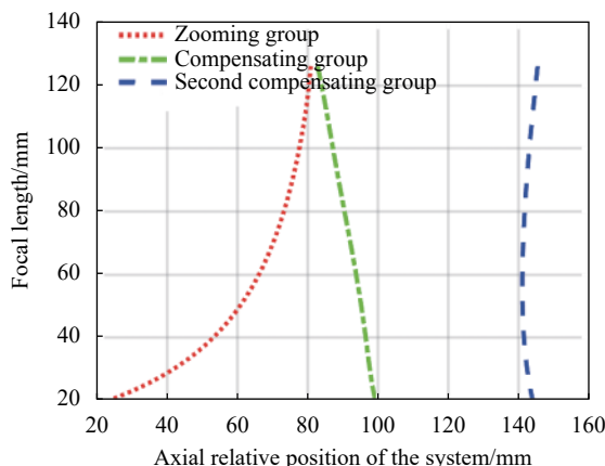
图 15 连续变焦光学系统凸轮曲线
