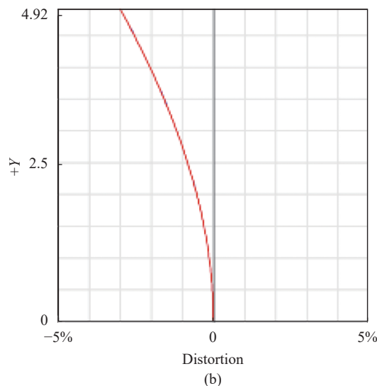
图 7 连续变焦光学系统小视场 (a) 及大视场 (b) 畸变情况
