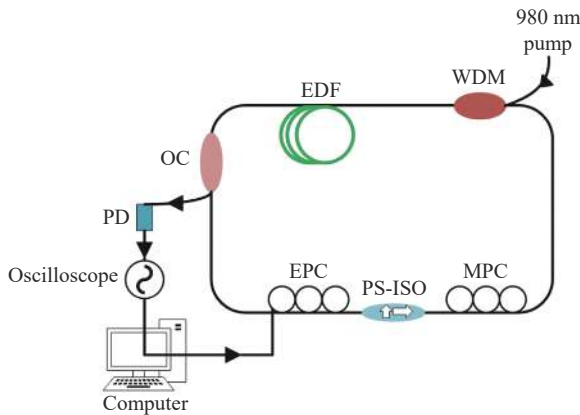
图 2 实验装置图
