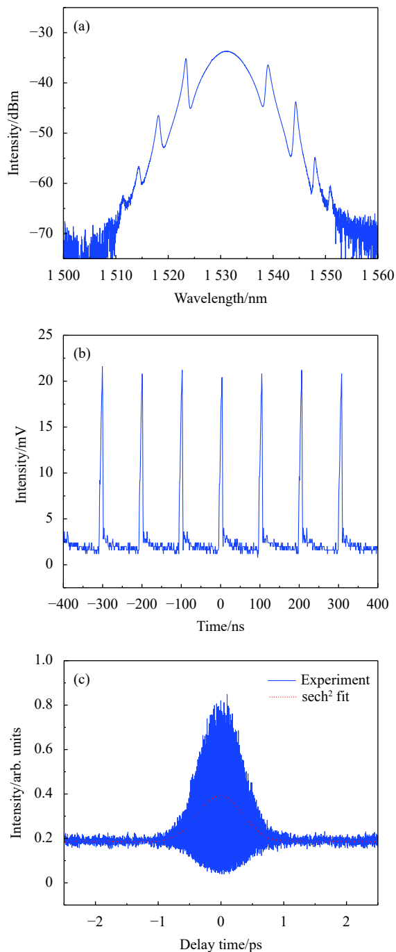
图 3 基频锁模孤子的 (a) 1531 nm 锁模态光谱图; (b) 1531 nm 锁模下的示波器曲线; (c) 1531 nm 锁模下的自相关谱图
