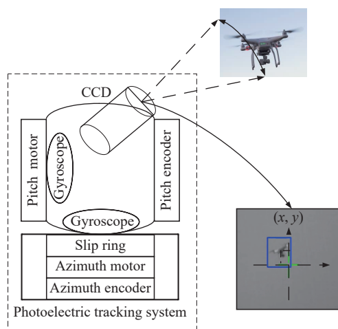
图 1 光电跟踪平台结构示意图
