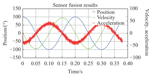
图 9 传感器融合结果
