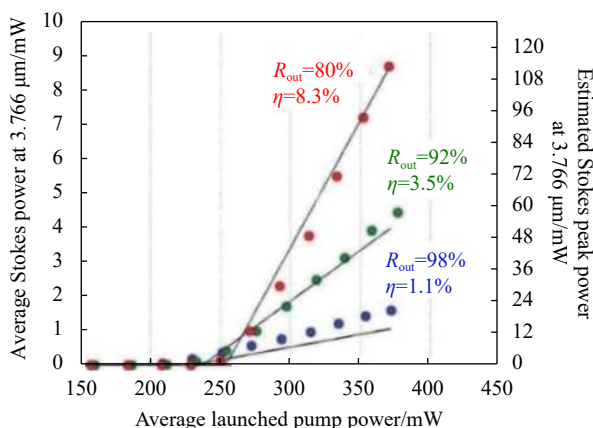
图 10 当输出端级联斯托克斯光栅的峰值反射率为 98%、92% 和 80% 时, 3.77 μm 拉曼激光的输出功率随泵浦功率的变化规律 [20]
