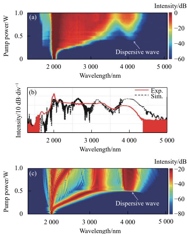
图 25 中红外色散波产生实验结果 [92] 。(a) 测量得 1 m 长氟碲酸盐玻璃光纤输出光谱随 1.98 μm 飞秒激光器平均泵浦功率的演化; (b) 平均泵浦功率 1 W 下的实验测量光谱与数值模拟光谱; (c) 数值模拟 1 m 长氟碲酸盐玻璃光纤输出光谱随 1.98 μm 飞秒激光器平均泵浦功率的演化
