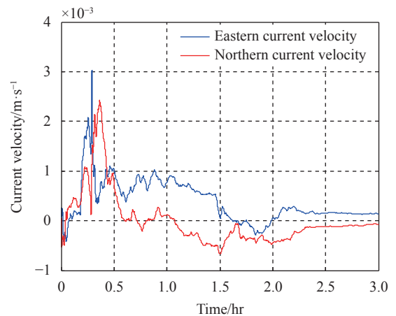
图 6 三次滤波后的洋流速度残差
