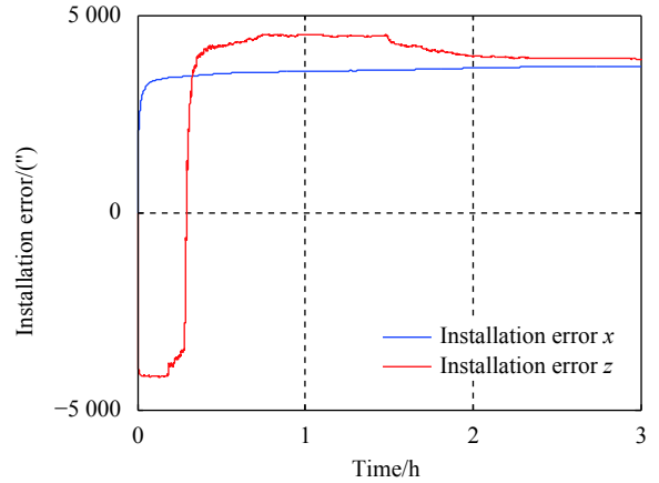
图 4 一次滤波后的安装误差角估计结果
