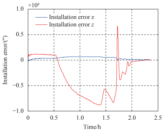
图 11 带里程仪的海上安装误差角估计残差
