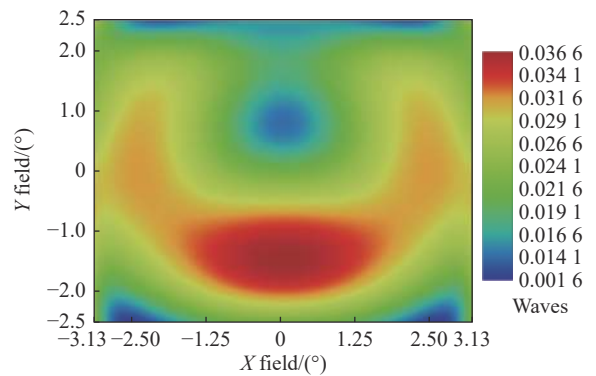
图 7 全视场 RMS 波像差分布
