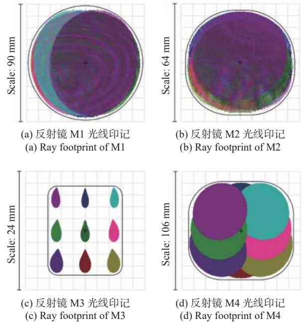
图 3 反射镜 M1~M4 光线印记 (不同颜色代表不同视场)
