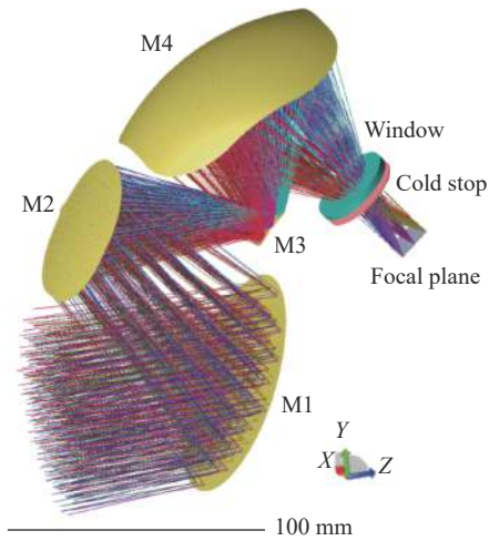
图 2 光学系统光路结构
