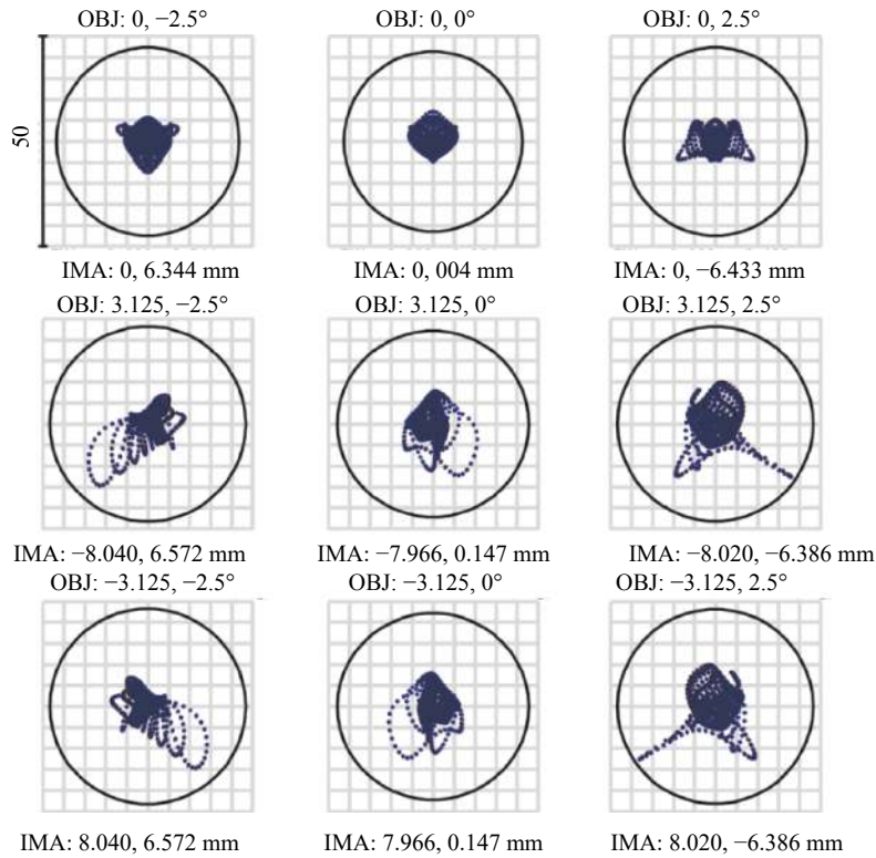
图 5 光学系统点列图
