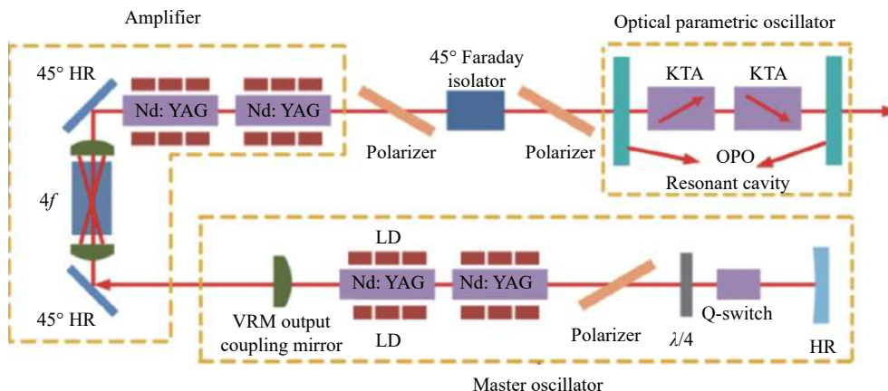
图 13 100 Hz 的高能量 KTA-OPO 实验装置图 [70]
