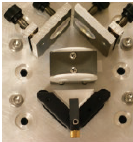
图 11 环形腔 KTA-OPO 的实物图 [67]
