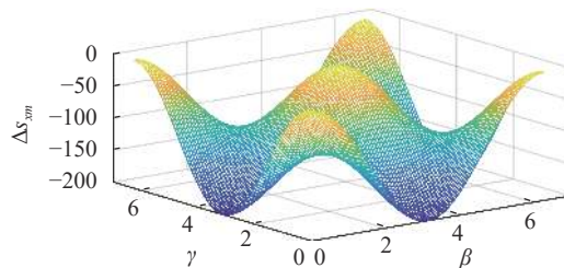
图 3 位移量为 100 mm 时的模拟测量误差
